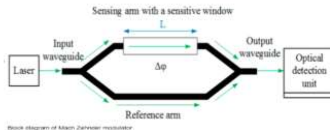
Fig 2. Mach Zehnder Modulator
